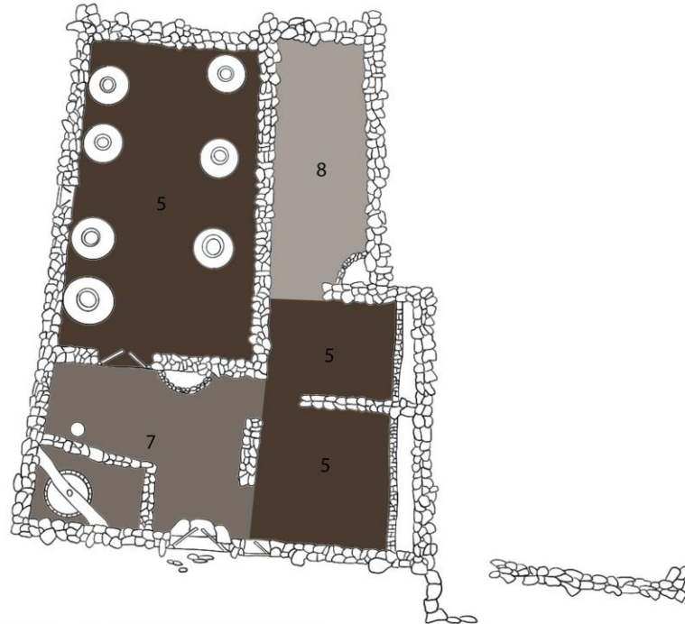
Οικία Αχιλλέα Δημήτρη. Κάτοψη ισογείου
